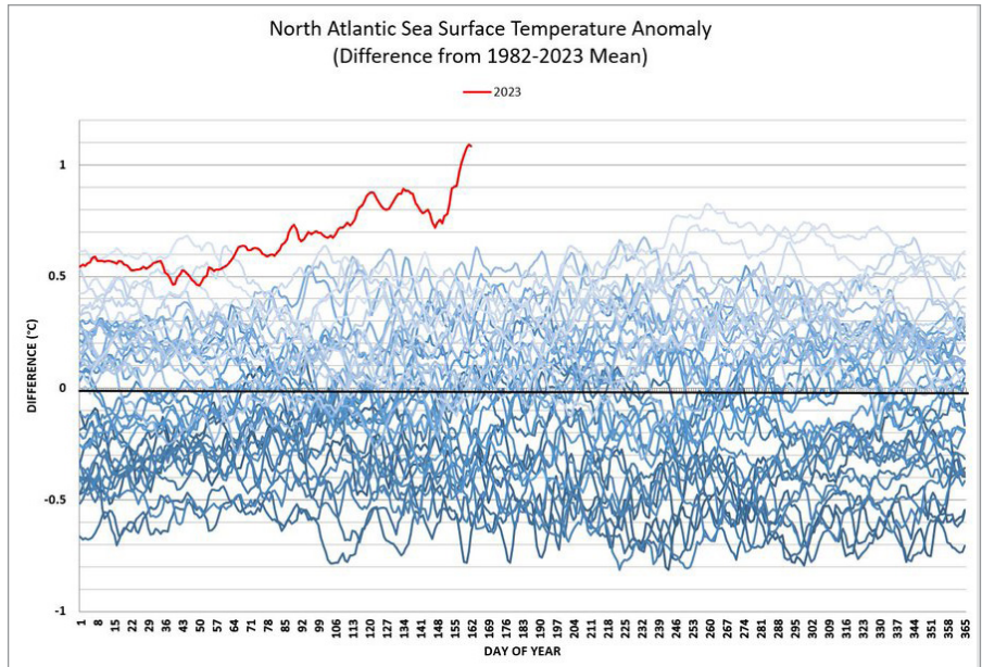
Die von Eliot Jacobson auf Twitter geteilte Grafik zur Oberflächentemperatur des Nordatlantik. Quelle: https://twitter.com/EliotJacobson/status/1668271214882615298
